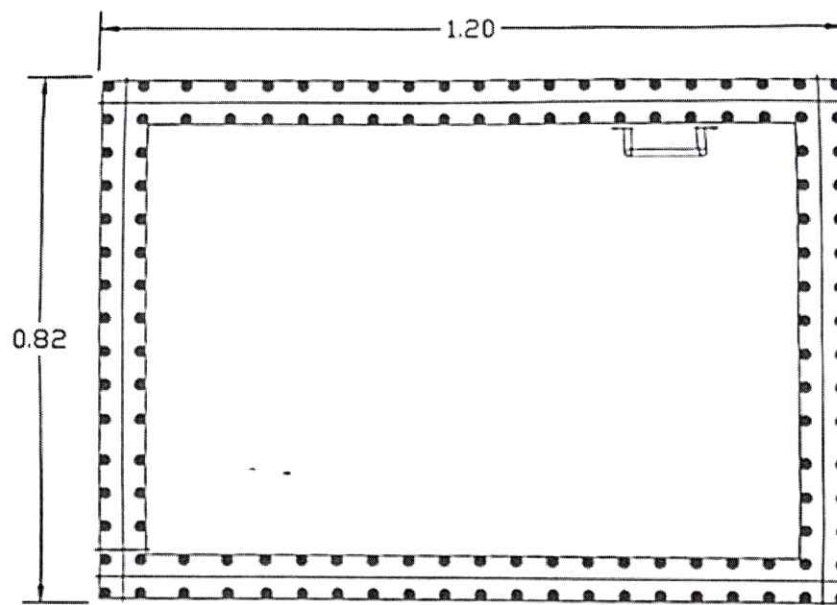
Planimetría presentada - Detalles de Caja proyectada (Estructura proyectada por parte de la entidad encargada)
