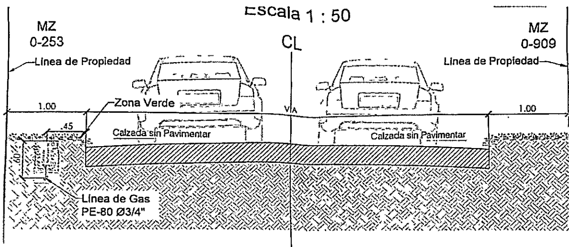
Planimetría presentada - Detalles de Instalación y excavación de tubería (Recorrido proyectado por parte de la entidad encargada)
