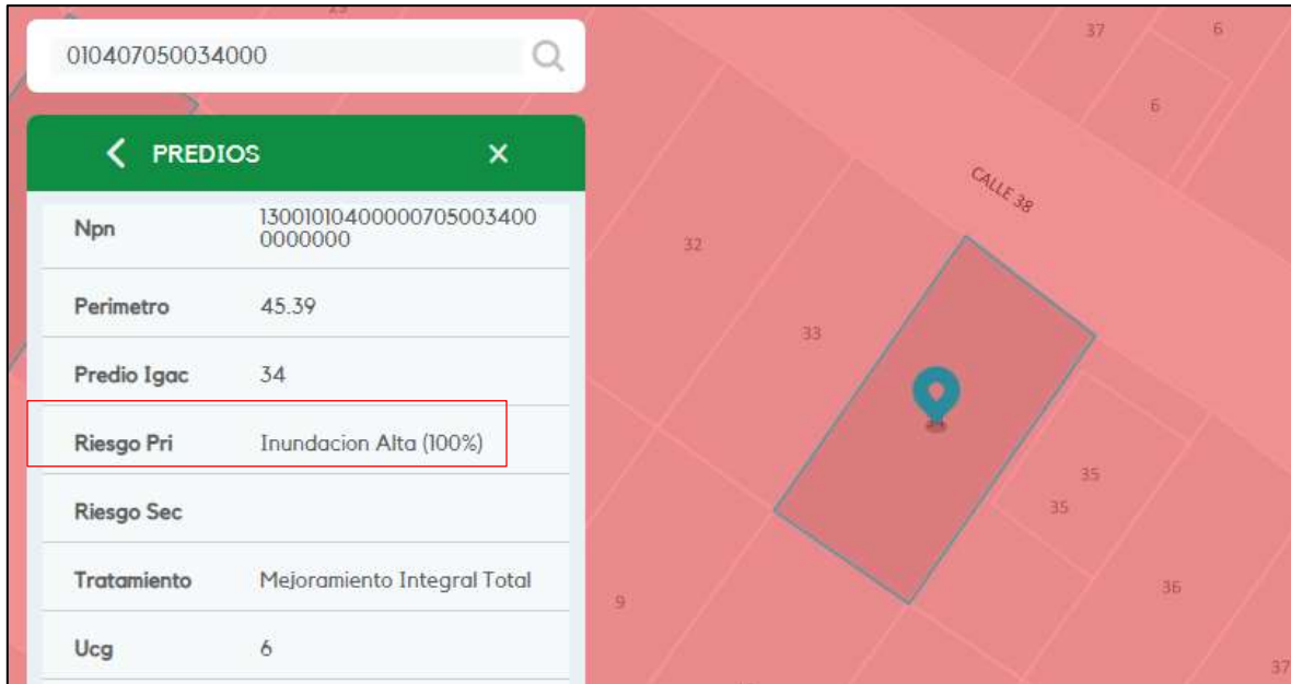
Ilustración 1. Plano de Susceptibilidad de Riesgos PDU 5B/7
