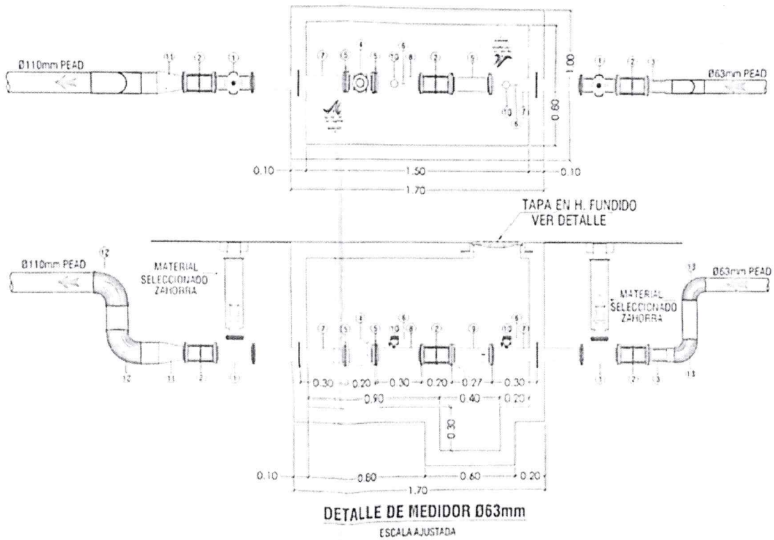
Planimetría presentada - Planta General - Detalles de Instalación y excavación de tubería
