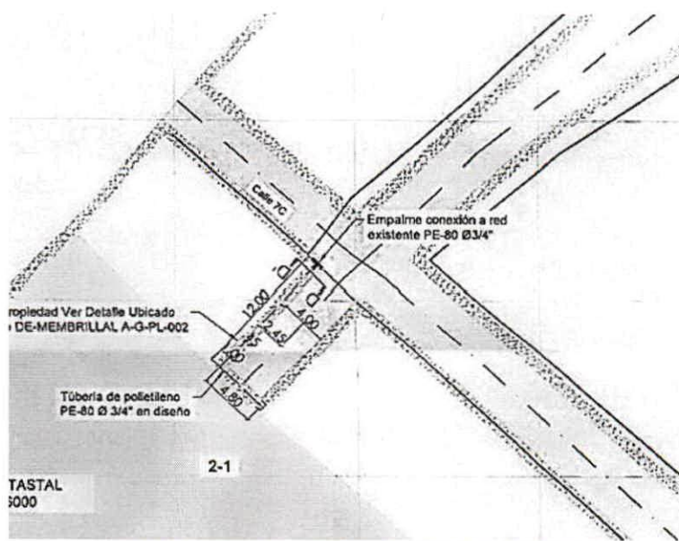
Planimetría presentada - Instalación y excavación de tubería
