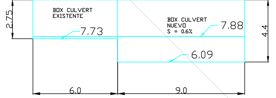
SECCION AGUAS ARRIBA (ALTERNATIVAS 1)
