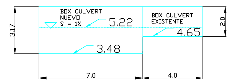
SECCION AGUAS ARRIBA (ALTERNATIVA 1)
